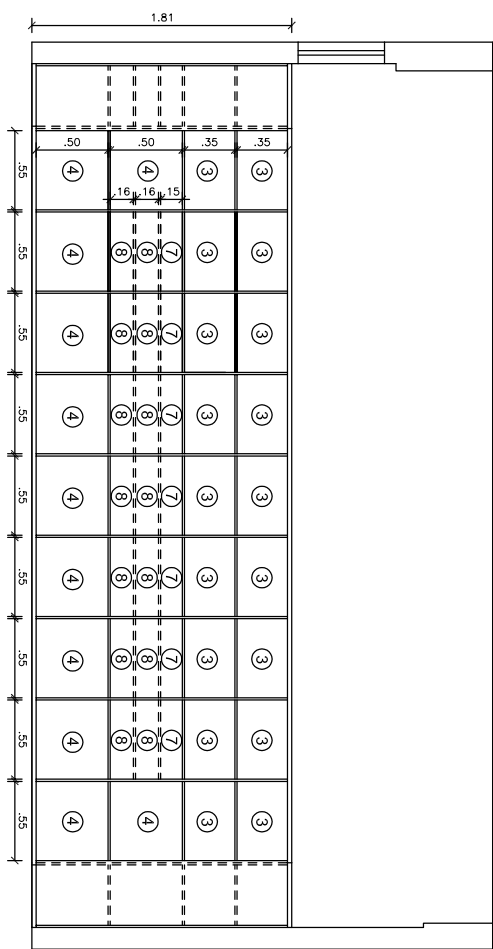
CORTE BB'
