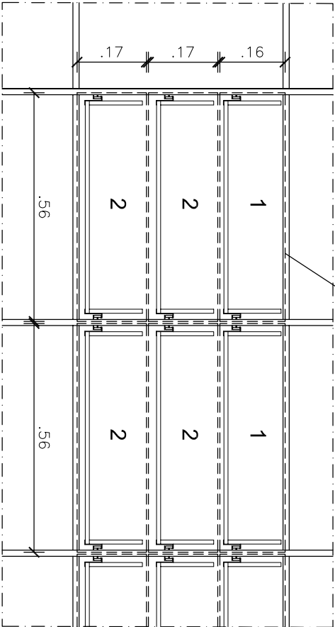
DETALHE GAVETAS - RECORTE NA VISTA A
