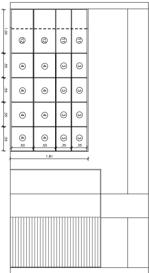
CORTE CC'
