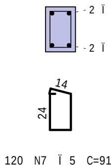
Corte A
