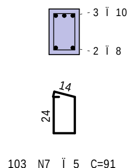
Corte A
