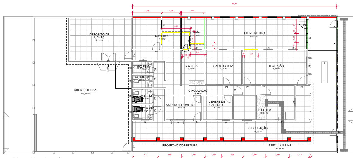
1 Planta Demolir e Construir 1 : 75
