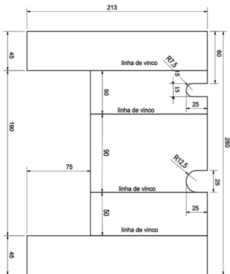
Figura 11 – Acessório – Cinta da caixa
