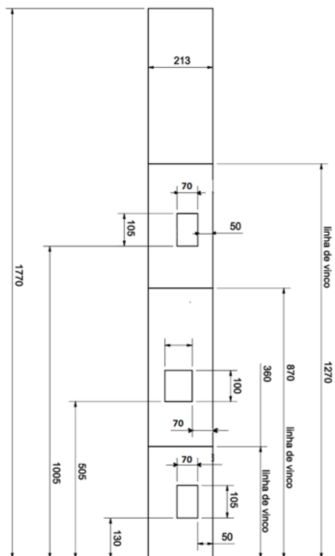
Figura 11 – Acessório – Cinta da caixa
