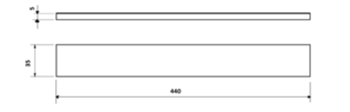
Figura 20 – Calço interno do nicho que apoia o cabo do terminal do mesário para todas as urnas, identificado como “D” na Foto 8 do Anexo I-II
