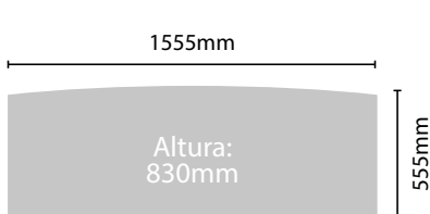
ARMÁRIO CREDENZA
